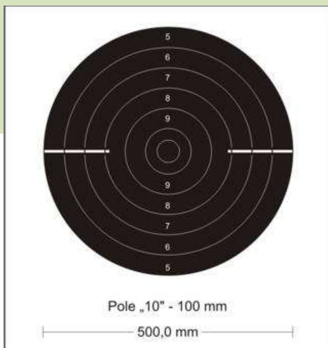
Tarcza do strzelań na 25 m w konkurencji pistolet sportowy-część szybka, pistolet centralnego zapłonu-część szybka i pistolet szybkostrzelny
