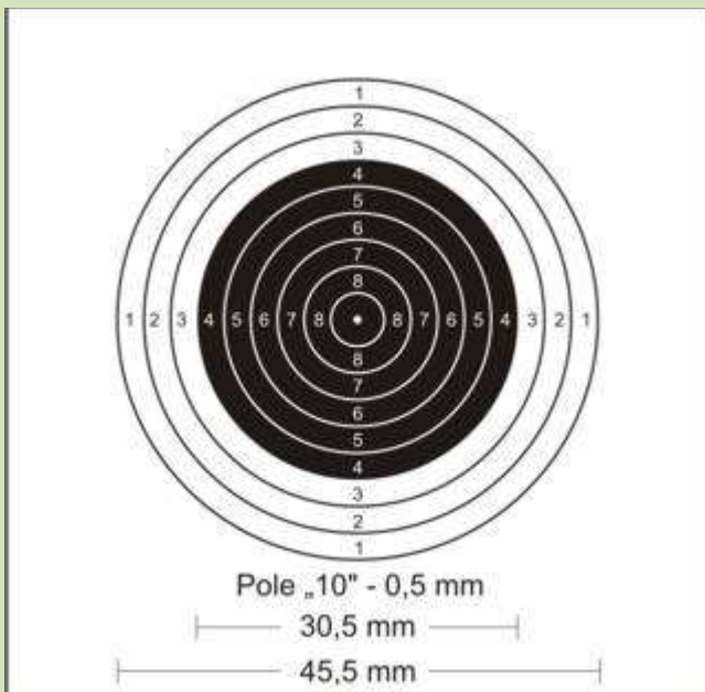
Tarcza do strzelań z karabinu pneumatycznego Odległość strzelania 10 m
